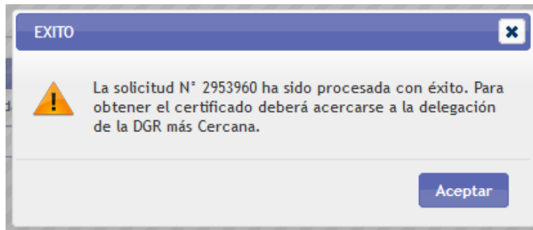
Figura 10. Mensaje Éxito.
